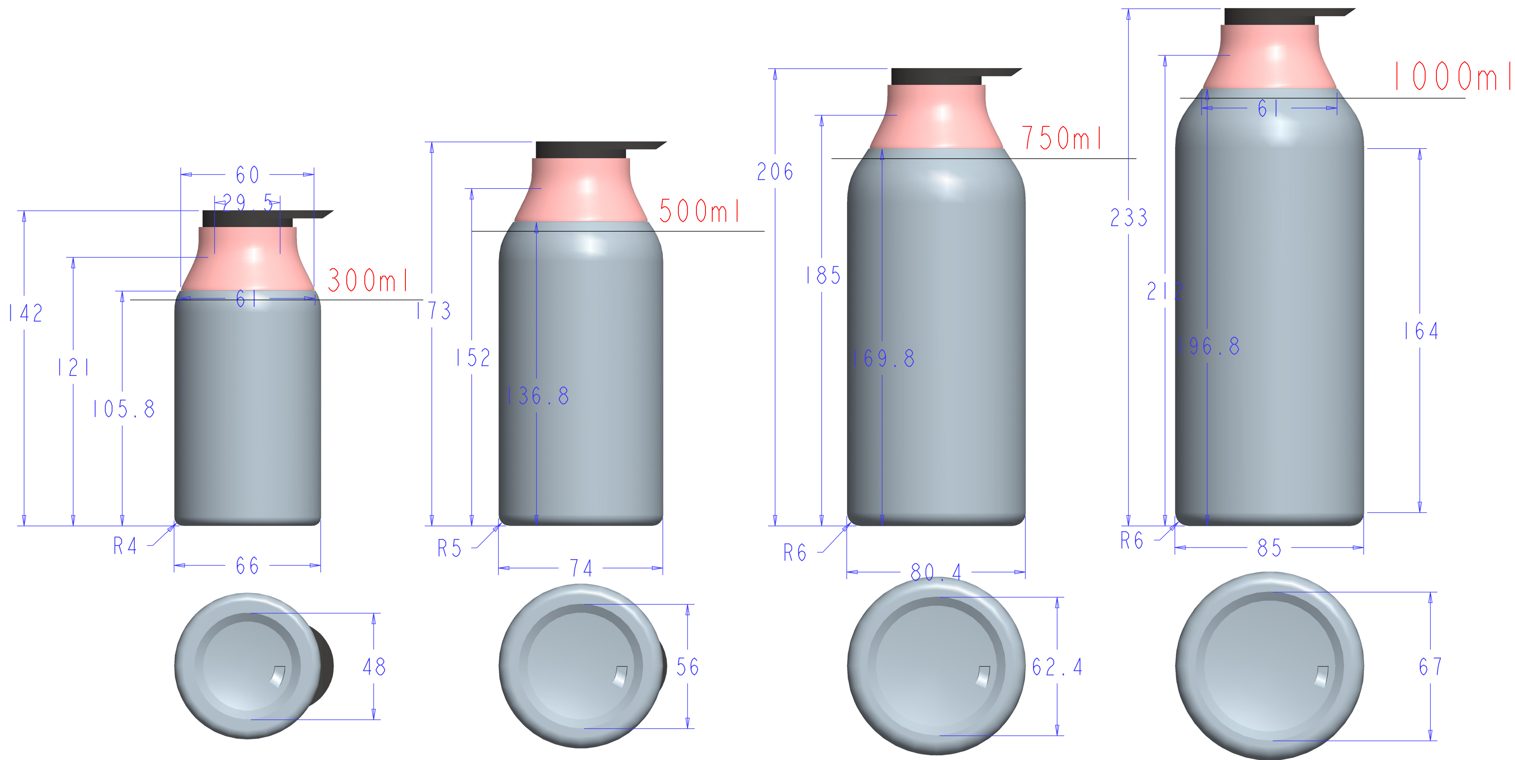
500ml | 设计瓶 瓶重55克32牙 满口容量540ml \pm 6ml 尺寸单位 mm
